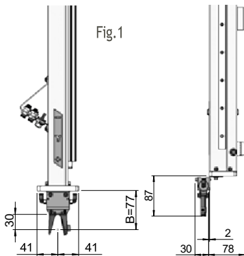
Standardversion mit Angusszange
